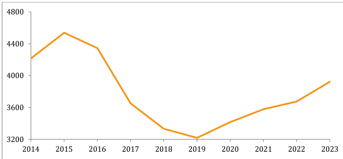
Schaubild 3 Absolute Militärausgaben, Trend 2014 – 2023 in Mio. USD
